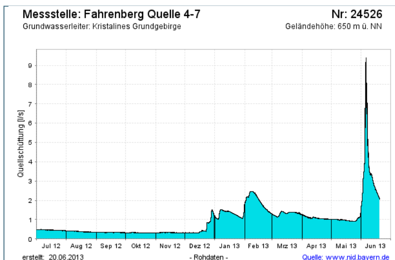
Abb. 6-3: Quellschüttung Fahrenberg 4-7 Gemeinde: Waldthurn, Landkreis: Neustadt a. d. Waldnaab (Oberpfalz) Messdaten seit 14.02.2011
