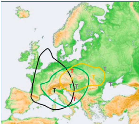
Abb. 1-1: Luftdruckstrukturen in 5,5 km Höhe. Tiefdruckzentren am 30. und 31.05. sowie am 01., 02. und 03.06.2013. Isolinie 552 gpm am 30. und 31.05. sowie am 01.06.2013. Am 02. und 03.06.2013 lag das 500 hPa-Niveau über 552 gpm und daher ist keine Isolinie zu sehen.
